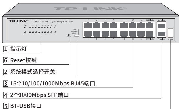
图1-4 TL-NS620-16GP2F前面板示意图
